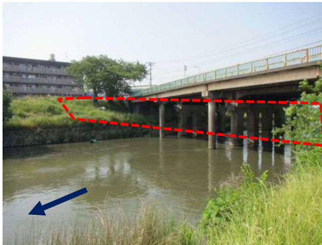
②-2五条川：清洲橋（県道西清洲線）仮橋工事
